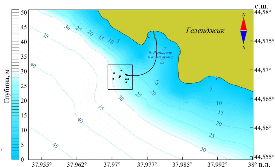
Рис. 22. – Схема расположения термокос в акватории Голубой бухты по данным работы [11] (воспроизведено по: Очередник, Зацепин, 2023). Кружки – точки постановки термокос; глубина в точках постановки 22–23 м. Расположение соответствует полигону настоящего исследования.
