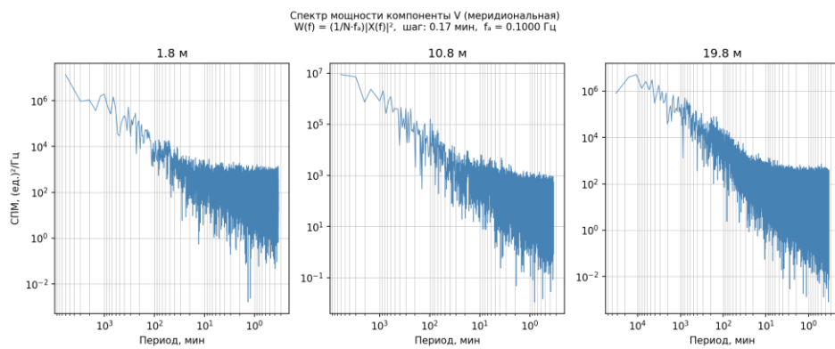
Рис. 16. – Спектры мощности меридиональной компоненты V для горизонтов 1,8; 10,8; 19,8 м. Периодограмма, ось периодов – минуты.
