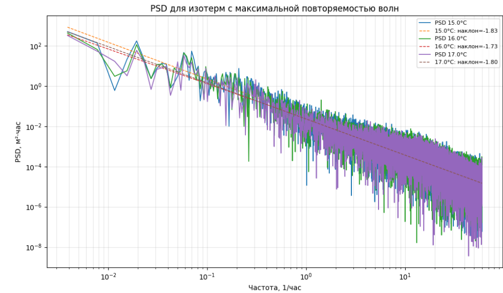
Рис. 20. – Спектральная плотность мощности (PSD) для изотерм 15,0; 16,0; 17,0 °C (наибольшая повторяемость волн). Пунктирными линиями показаны линейные аппроксимации наклона.
