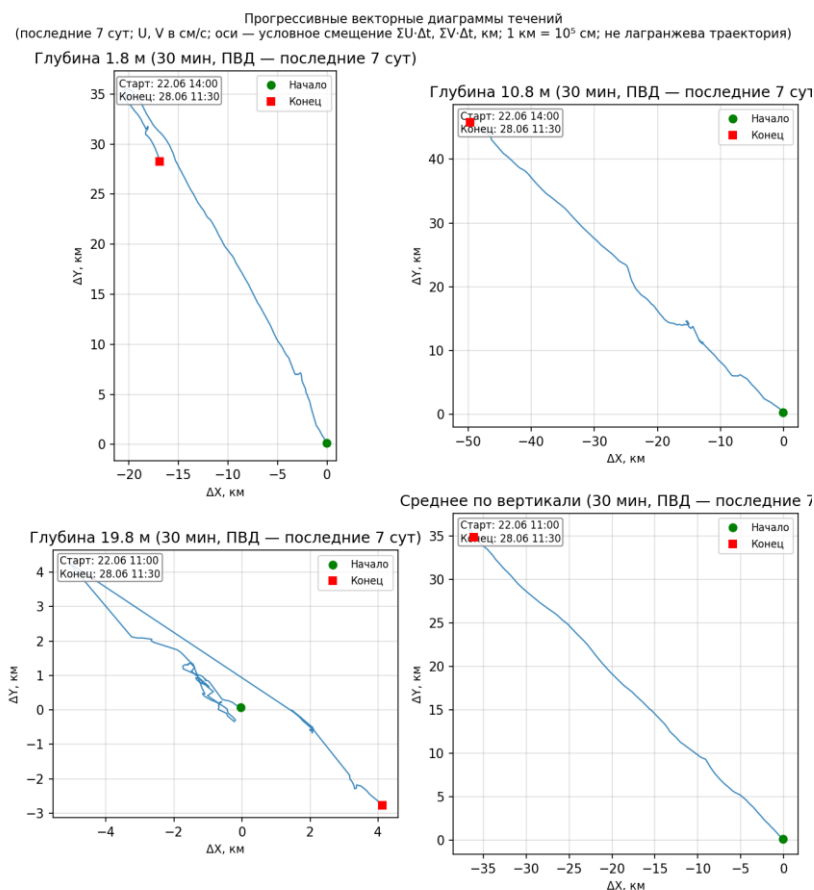
Рис. 17. — Прогрессивные векторные диаграммы течений ( X = \Sigma U \cdot \Delta t , Y = \Sigma V \cdot \Delta t ) для горизонтов 1,8; 10,8; 19,8 м и вертикального среднего. Начало — зелёный маркер, конец — красный.
