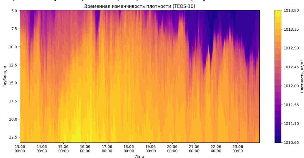
Рис. 2. – Поле временной изменчивости плотности.
