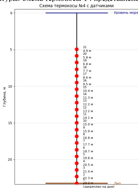
Рис. 4. – Схема термокосы Т4 с отмеченными датчиками (красный) и их медианными глубинами.
