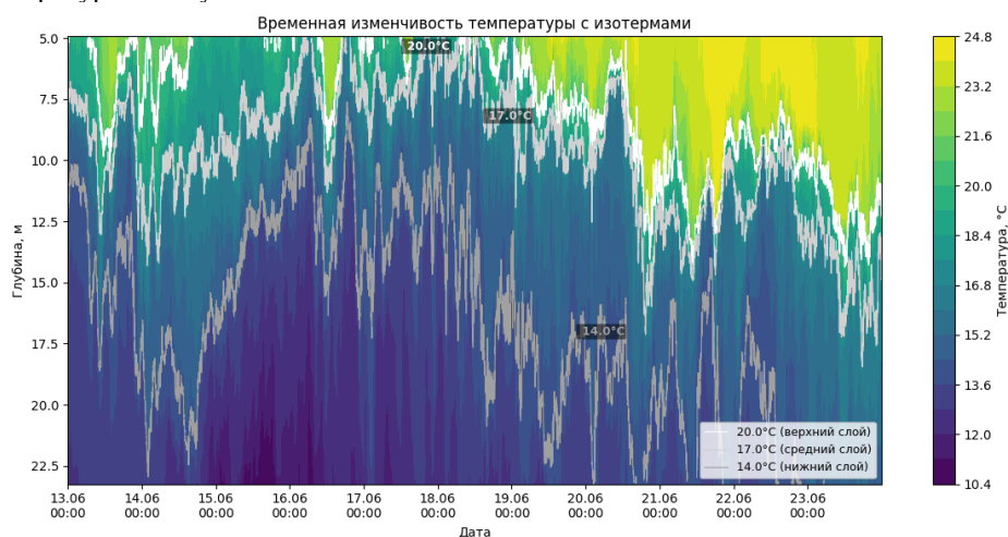
Рис. 6. – Временные колебания изотерм 14°C, 17°C, 20°C.
