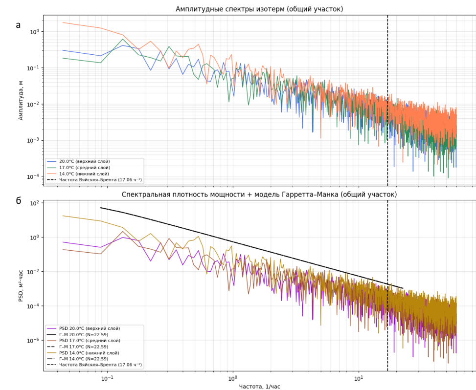
Рис. 8. – Результаты спектрального анализа вертикальных смещений изотерм на общем непрерывном участке (22,6 ч): а – амплитудные спектры (FFT) для изотерм 14, 17 и 20 °C; б – спектральная плотность мощности (PSD) для тех же изотерм (цветные
