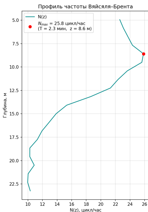
Рис. 3. – Профиль частоты Вайсяля–Брента с указанным максимальным значением 25.8 цикл/час, период T = 2.3 мин.
