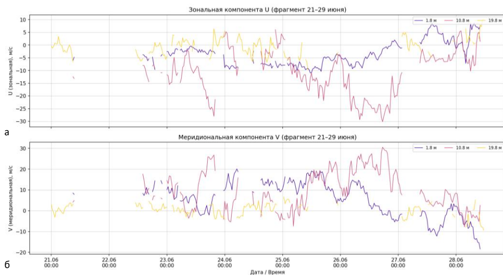
Рис. 13. – Временные ряды компонент скорости U (а) и V(б) на горизонтах 1.8 и 10.8 м в период 21–29 июня 2023 г. (укрупнённый фрагмент). Данные за 9–21 июня на указанных горизонтах отсутствуют.
