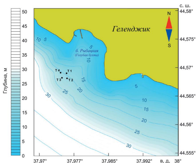
Рис. 1 – Положение заякоренных термокос на карте батиметрии [6].
